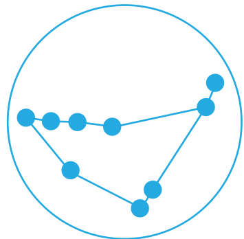
Capricornio
