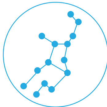
Virgo
