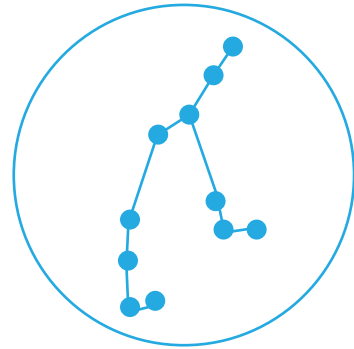
Perseo
