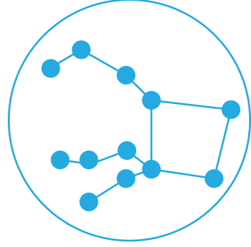
Pegaso
