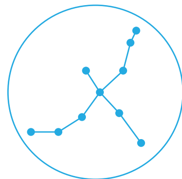
El cisne
