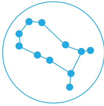
Géminis
