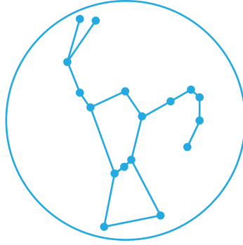
Orión
