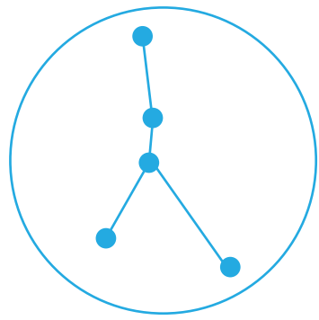
Cáncer
