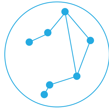
Libra
